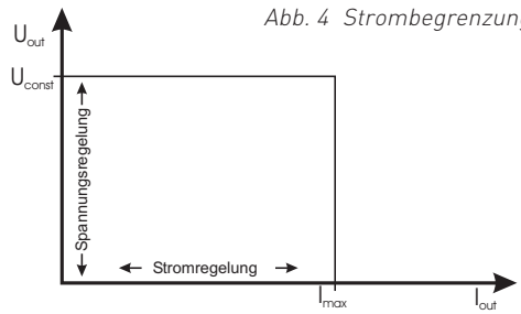
Abb. 4 Strombegrenzung
