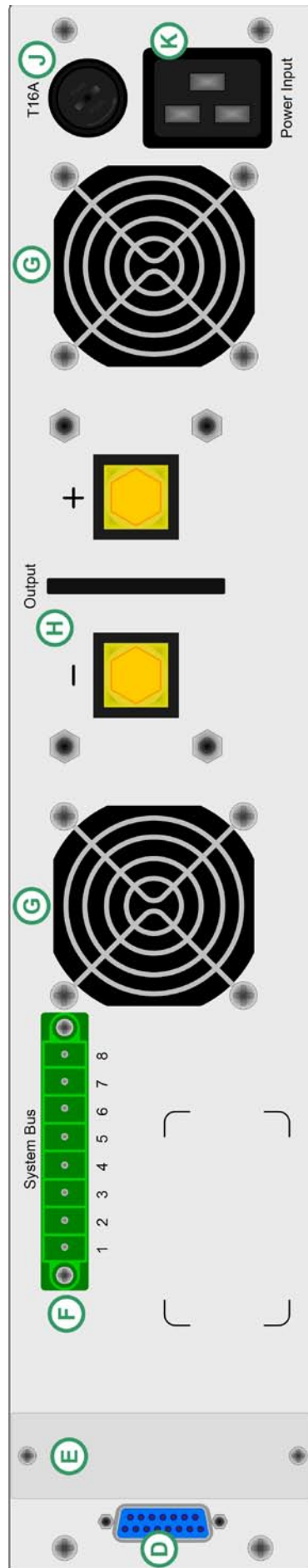
Bild 2. Rückansicht
