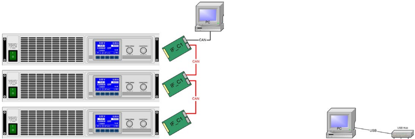
Bild 7. CAN-Vernetzungsbeispiel, gilt auch für GPIB
