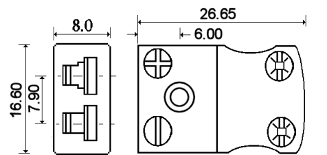
Miniature Socket
