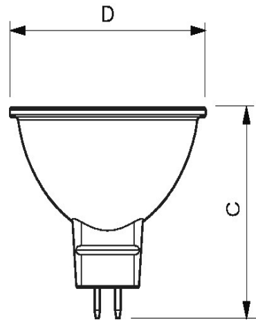
Abmessungsskizze
