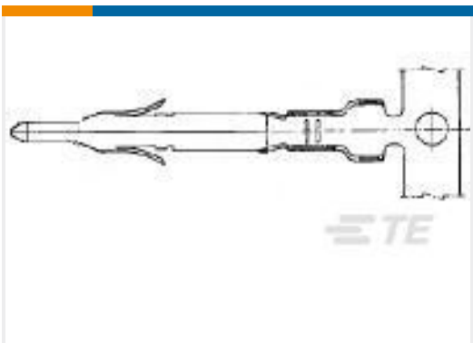
TE Part #170363-1 MINI UNIVERSAL M-N-L PIN LP
