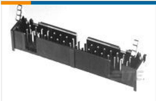
TE Part #1-1761606-0 IDC LOW PRO HDR 30P VERT LG LA
