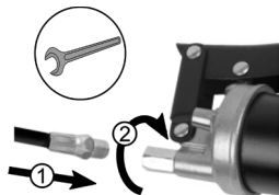
Figura 2: Collegamento del tubo flessibile
