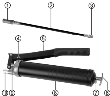
Figure 1 : Vue d'ensemble
