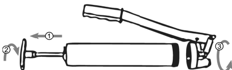
Bild 3: Pressenkopf abschrauben
