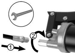
Bild 2: Schlauch anschließen
