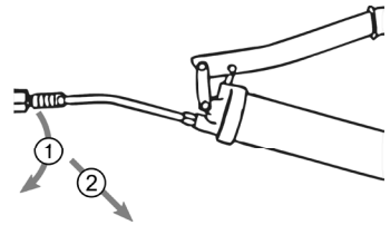
Bild 11: Schmiernippel lösen
