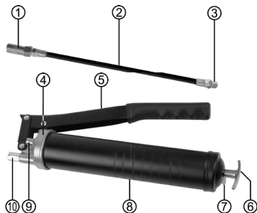
Figura 1: Schema
