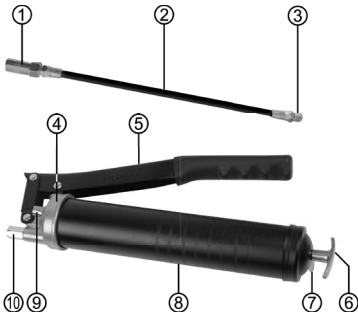
Bild 1: Übersicht
