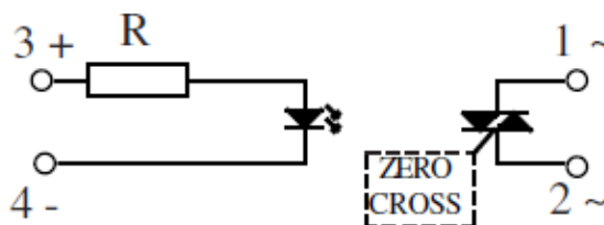
schéma équivalent / Equivalent circuit
