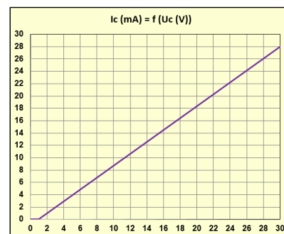
fig. 1 :Control characteristic / Caractéristique d'entrée
