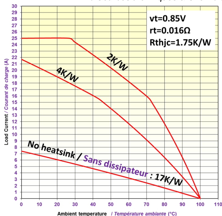
Fig. 2 Thermal curves and heatsink choice / Courbes thermiques & Choix dissipateur thermique /
