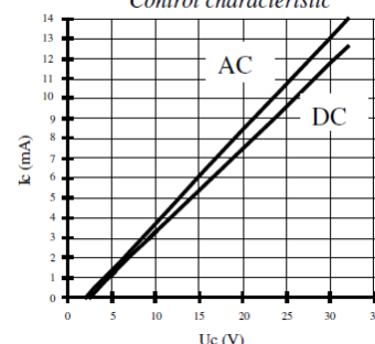
Fig. 1 :Caractéristique d'entrée / Control characteristic
