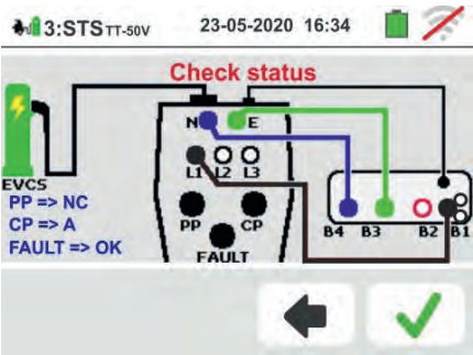
Anschlusschema für Status A im Prüfablauf EVSE
