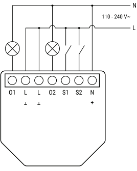
Fig. 1. Dual-channel switch, 110-240 V~ power supply Abb. 1. Zwei-Kanal-Schalter, 110-240 V~ Spannungsversorgung Fig. 1. Interruttore a due canali, alimentato a 110-240 V~
