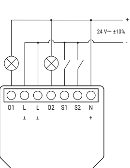
Fig. 2. Interruptor / conmutador bicanal, alimentación de 24-30 V~
