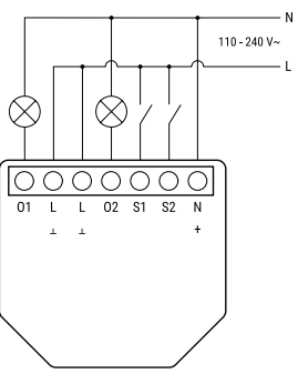
Fig. 1. Interruptor / conmutador bicanal, alimentación 110-240 V~
