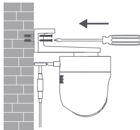
การติดตั้งขายึดติดผนัง
