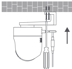
การติดตั้งขายึดติดเพดาน
