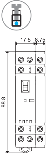
Typ 22.32 + 022.33/022.35 Käfigklemmen
