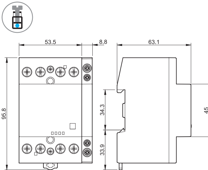
Typ 22.44/22.64 + 022.63/022.65 Käfigklemmen
