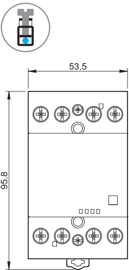
Typ 22.44/22.64 Käfigklemmen
