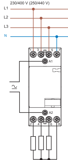
Typ 22.74
