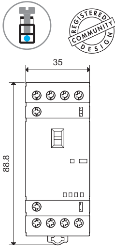
Typ 22.34 Käfigklemmen
