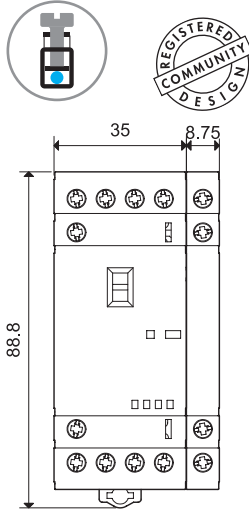
Typ 22.34 + 022.33/022.35 Käfigklemmen
