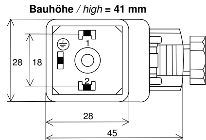
Kontaktanordnung bei Auslieferung Contact configuration by delivery
