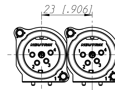
min. Einbauabstand min. assembling distance M 1:1
