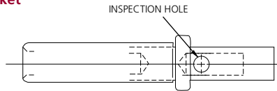
Socket
