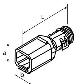
Receptacle 180°
