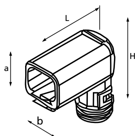
Receptacle 90°
