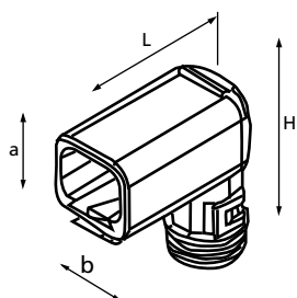
Receptacle 90°
