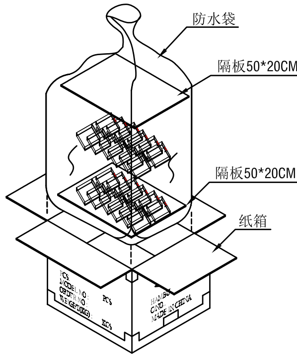
100PCS/CTN (580*230*230mm) 一排25pcs 上下兩排
