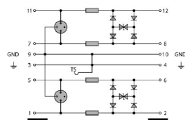
Complete module direct grounding, with remote signalling Komplettsmodul direkte Erdung, mit Fernmeldung
