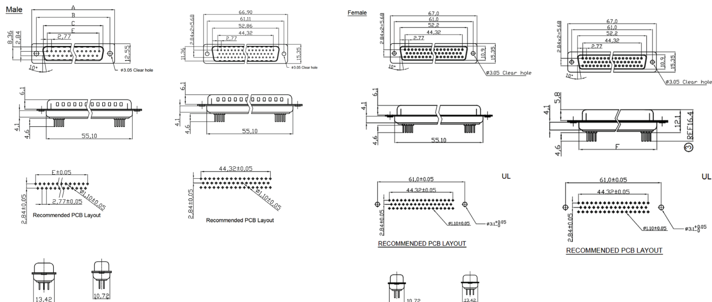
Dimensions
