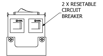
VIEW A-A
