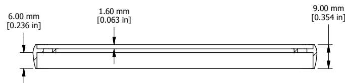
OPEN BEZEL
