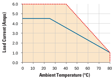
DRxxx06
