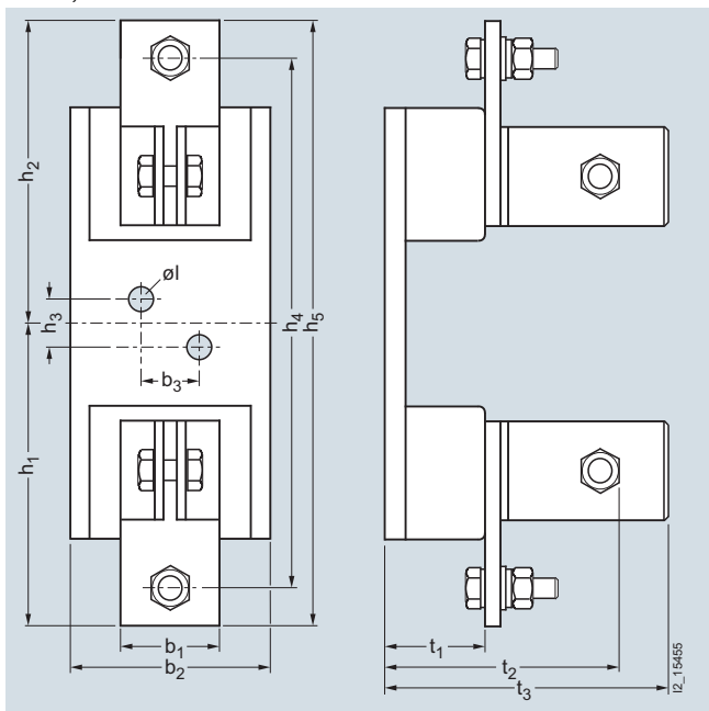
3NH3530
