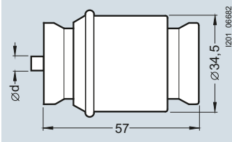
5SC1, 5SC2
