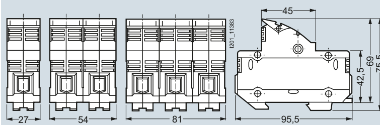
3NC149.
