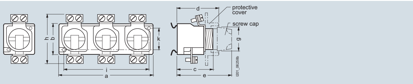
5SG15
