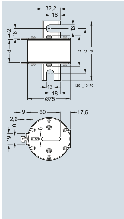
3NC34...-1
