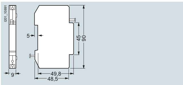
3NW7901 3NW7902
