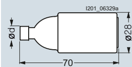
5SD6, 5SD8
