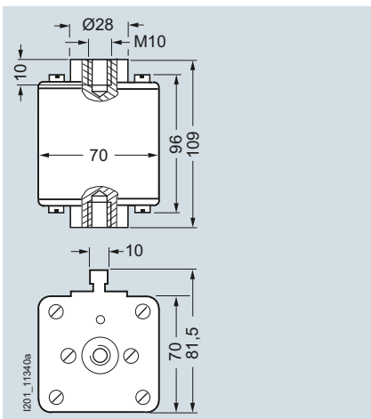
3NE3635-6
