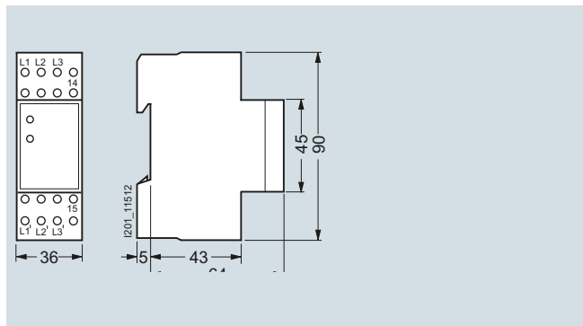
5TT3170
