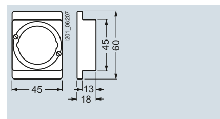
5SH5233 (A6)
