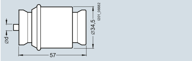
5SD510, 5SD520
