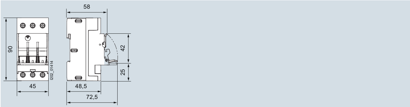
3NW703.-1 3NW753.-1HG
