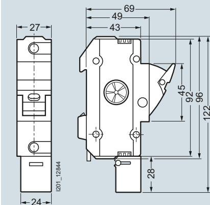
3NC1491-5
