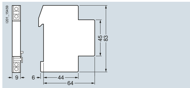
3NW7903
