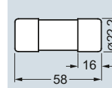
3NC22..
