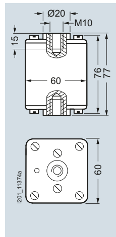
3NE43...-6B, 3NE4337-6
