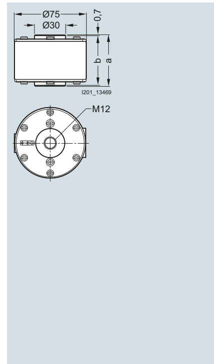
3NC34...-6
