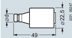
5SB1, 5SB2
