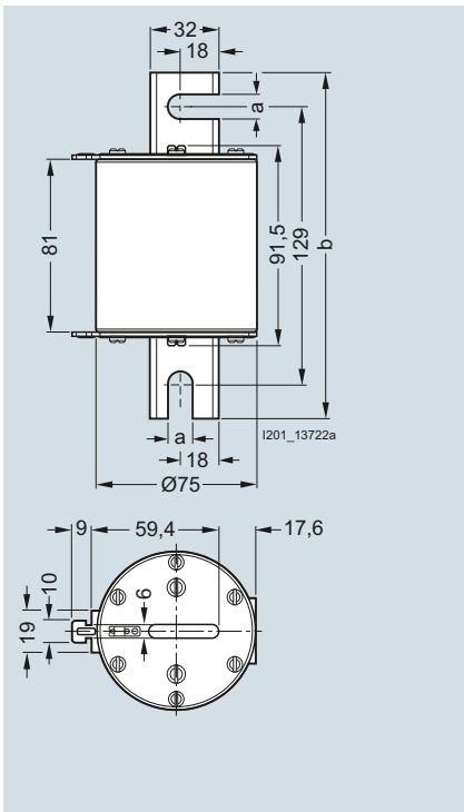
3NE3...-0C, 3NE36...-1C
