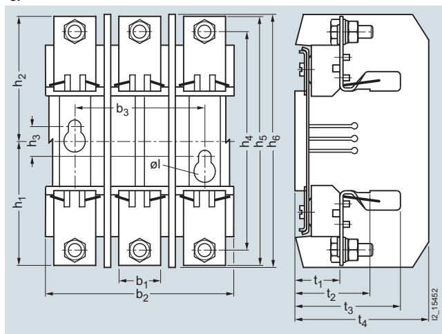
3NH4230
