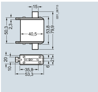
3NE18...-0
